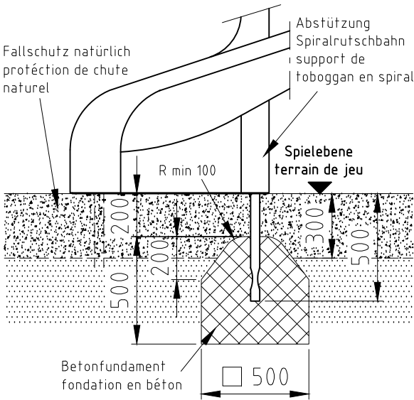
Fundament F11.1
