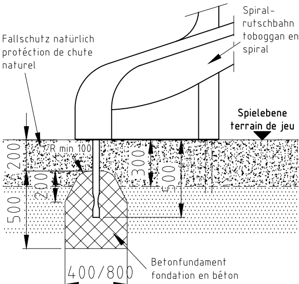
Fundament F11.
