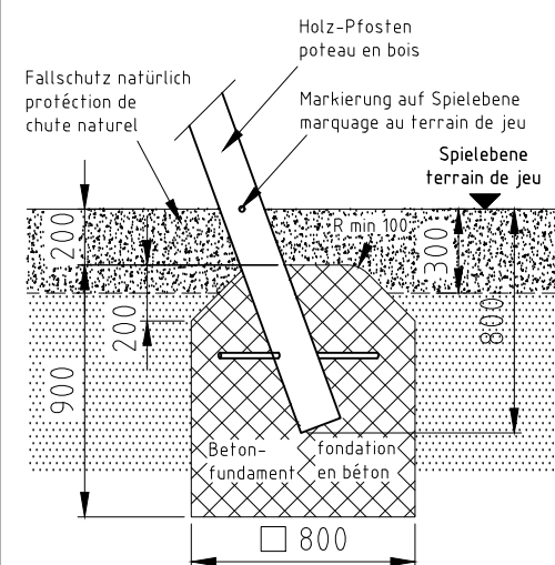
Fundament F91
