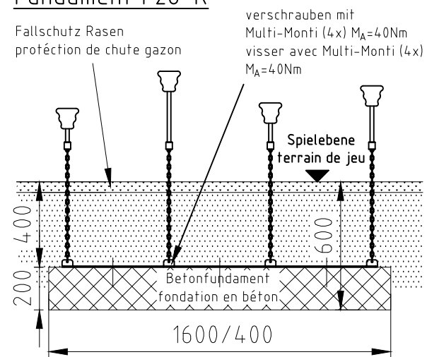
Fundament F26-R
