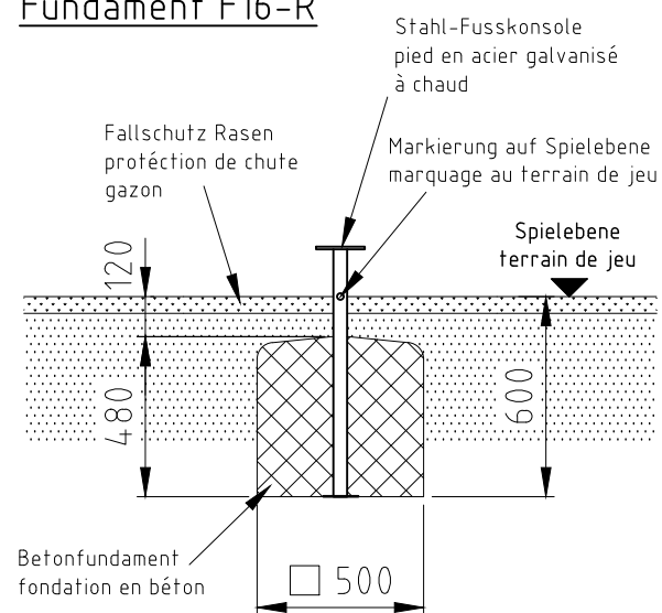
Fundament F16-R
