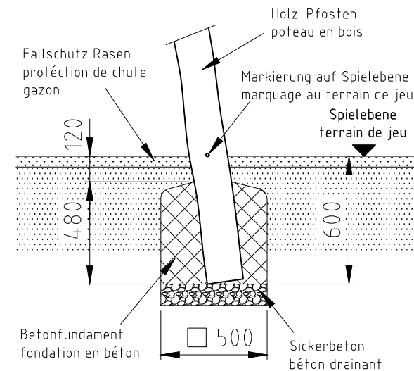
Fundament F16.1-R
