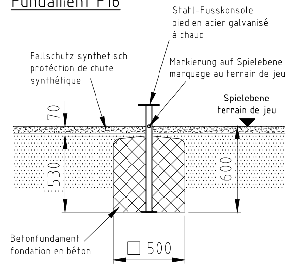
Fundament F16
