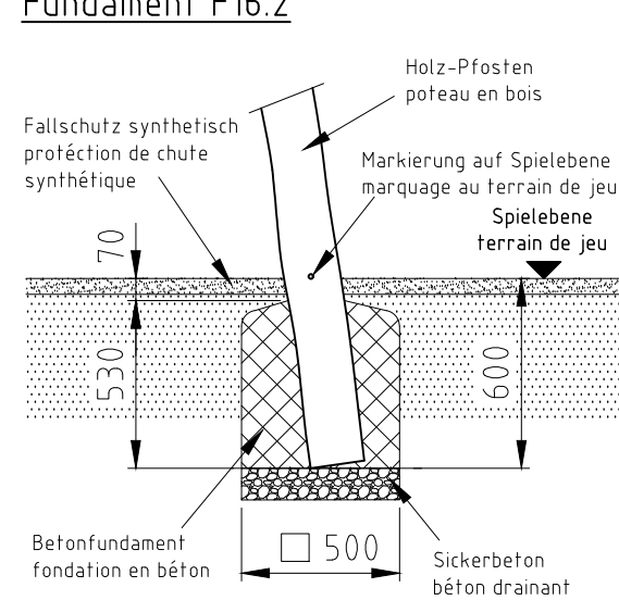
Fundament F16.2
