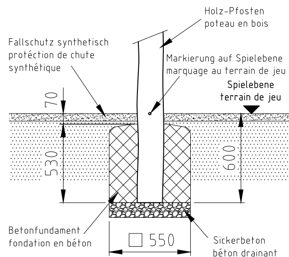
Fundament F01
