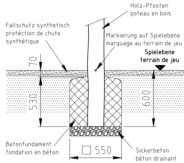
Fundament F01
