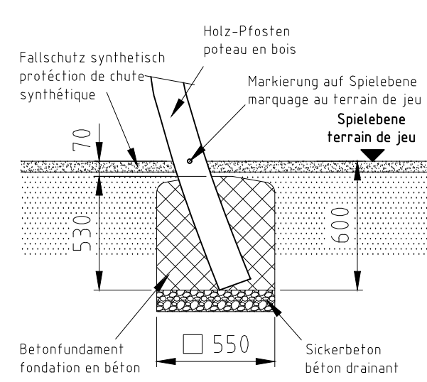
Fundament F31
