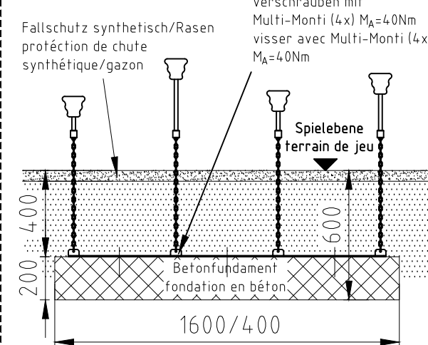
Fundament F26
