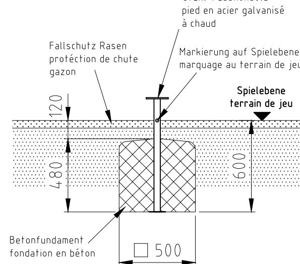
Fundament F16-R
