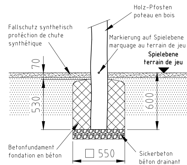
Fundament F01
