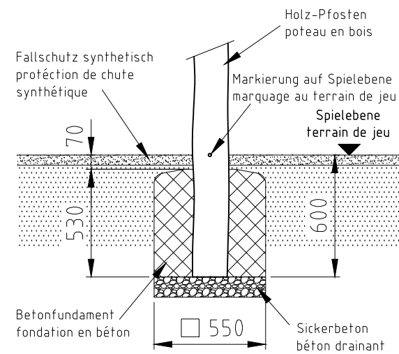
Fundament F01
