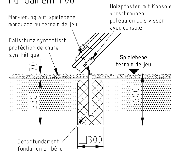
Fundament F06
