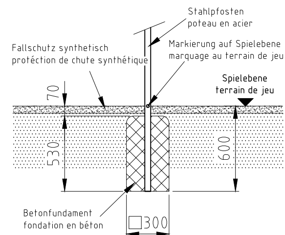
Fundament F20
