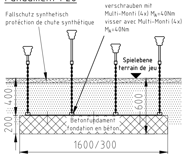
Fundament F26
