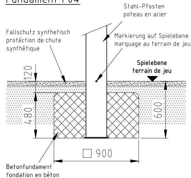
Fundament F04
