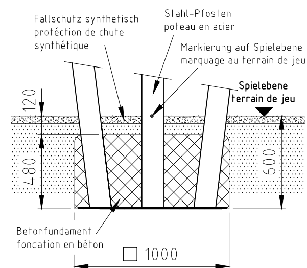
Fundament F01
