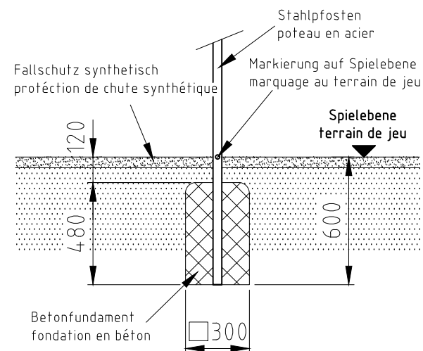
Fundament F20
