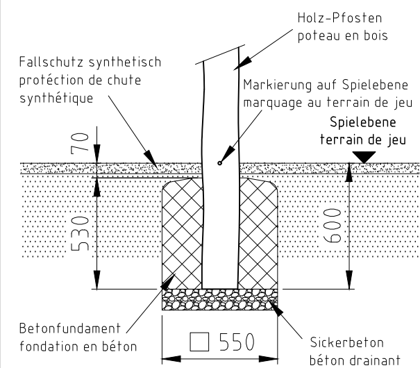
Fundament F01
