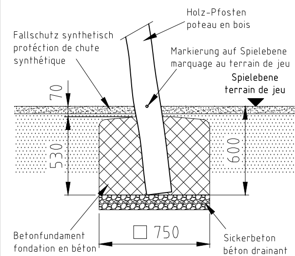
Fundament F06
