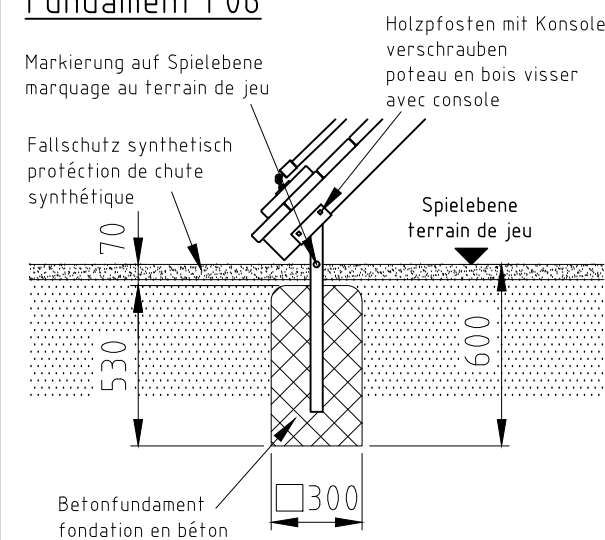
Fundament F06
