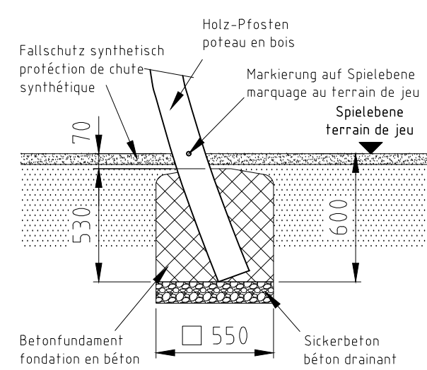
Fundament F31
